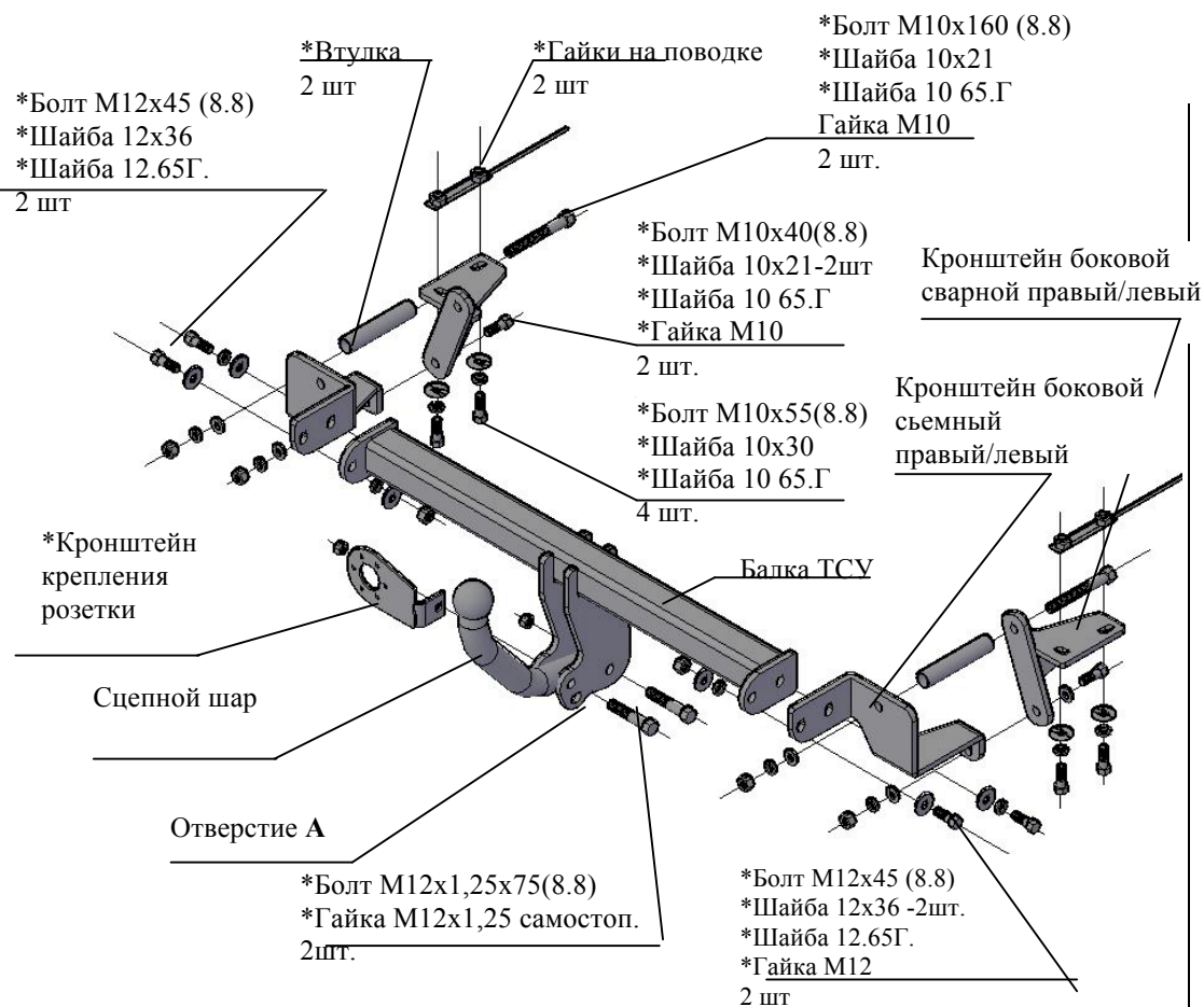
Рис.1 Тягово-сцепное устройство 9920
