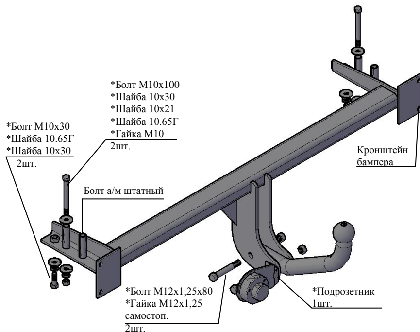
Рис.1 Тягово-сцепное устройство 9420
