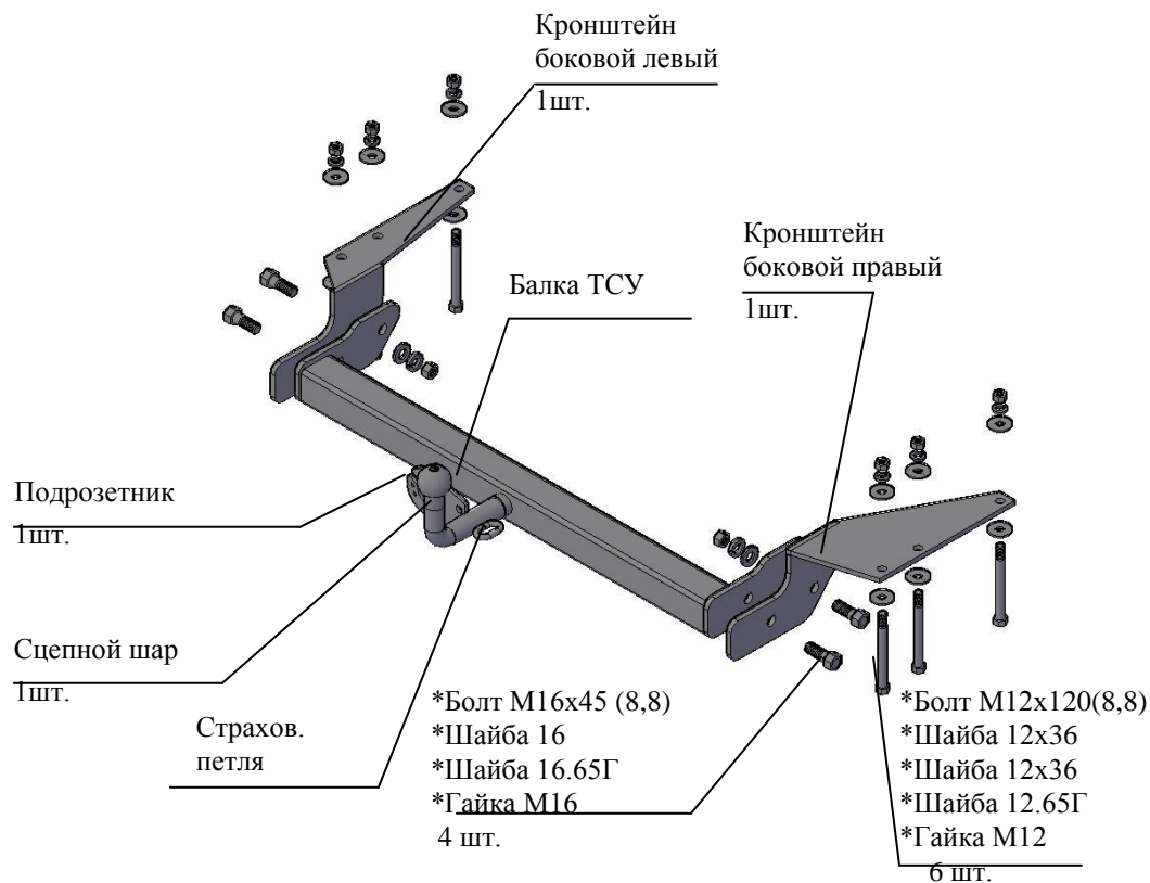
Рис.1 Тягово-сцепное устройство 7510 .
