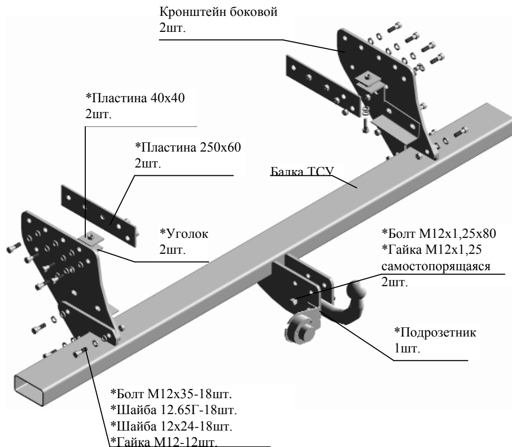
Рис.1 Тягово-цепное устройство 7110
